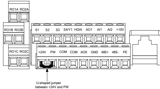
Рис. 4-34 Положение U-образной перемычки 3-фазного ПЧ 380 В 1,5–7,5 кВт
