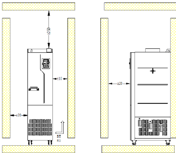
Рис. 4-7 Требования к монтажному пространству 43
