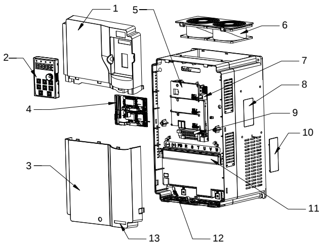
Рис. 3-5 Конструкция изделия
