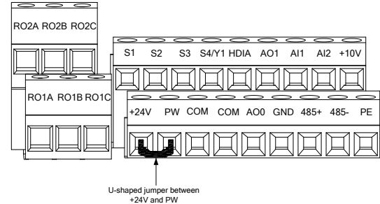
Рис. 4-35 Положение U-образной перемычки 3-фазного ПЧ 380 В 11–500 кВт
