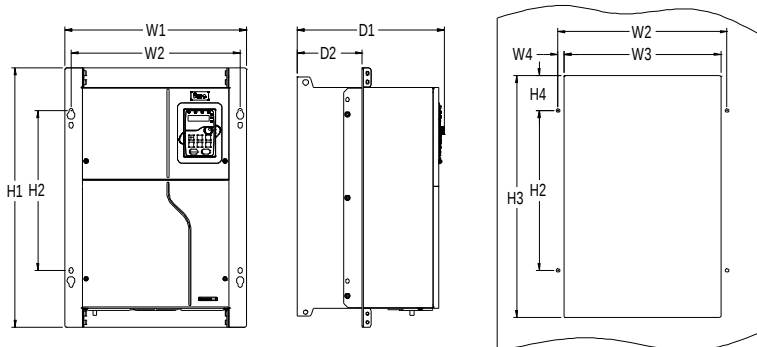
Рис. С-12 Чертеж для фланцевого монтажа моделей ПЧ 380 В 110–200 кВт
