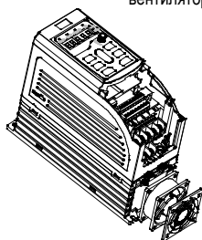
Рис.8-1 Обслуживание вентилятора для моделей 2,2–7,5 кВт (с помощью инструментов)
