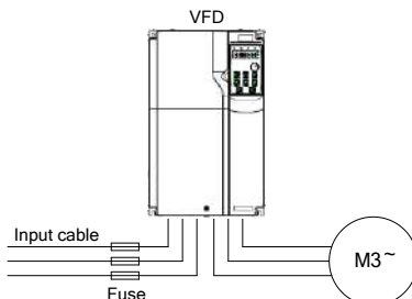
Рис. 4-39 Конфигурация предохранителя
