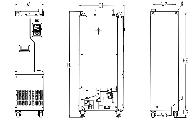
Рис. С-8 Чертеж для настенного монтажа моделей ПЧ 380 В 220–250 кВт
